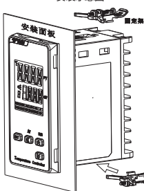
安装示意图
