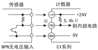
NPN无电压输入
