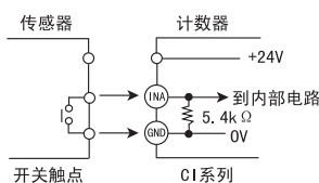
开关触点
