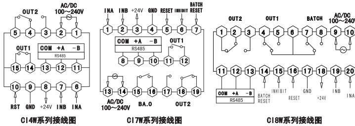
CI4W系列接线图
