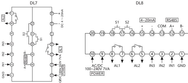
注: 接线如有变动, 以实际仪表机壳上的接线图为准
