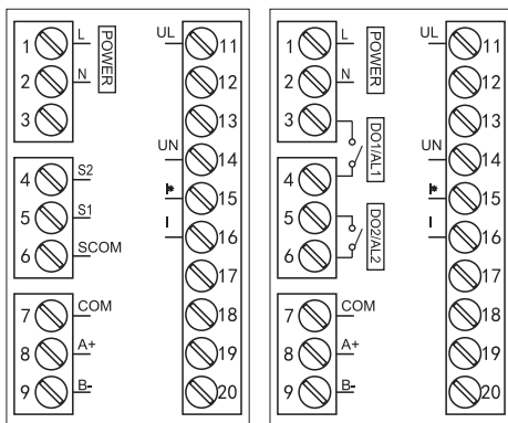
接线图请以实物机壳为主
